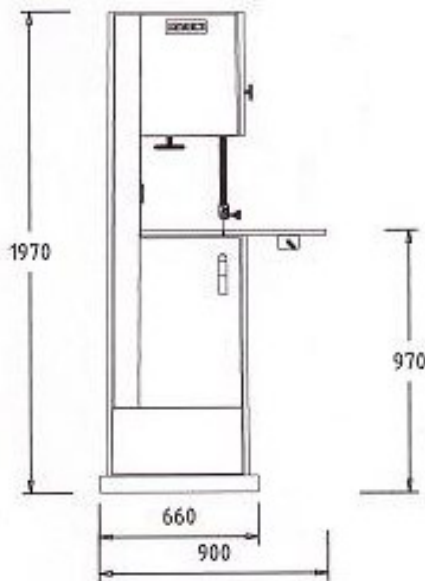
VISTA LATERAL
